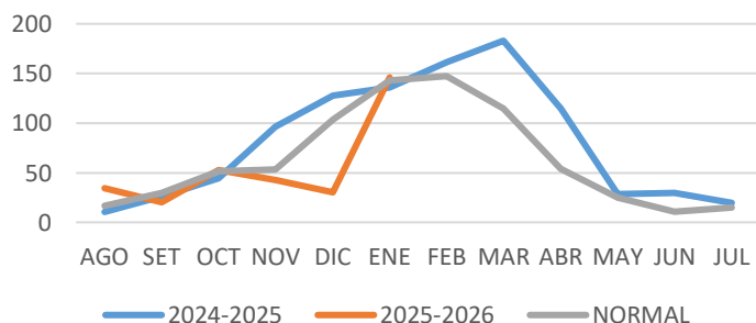
PRECIPITACION (mm) LIRCAY - ANGARAES (3,303 msnm)
