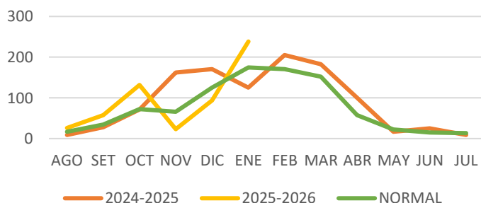
PRECIPITACION (mm) COLCABAMBA - TAYACAJA
