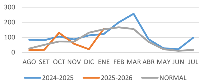
PRECIPITACION (mm) HUANCAVELICA
