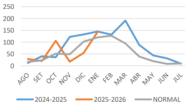
PRECIPITACION (mm) ACOBAMBA
